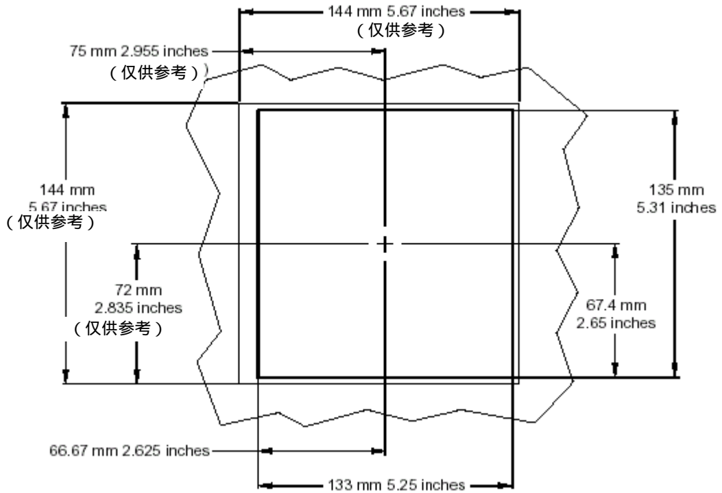
图 6 导线管开孔尺寸
